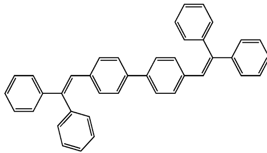
DPVBi
